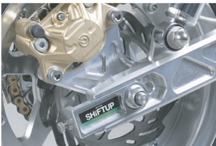
キャリパー上側への取り付け
