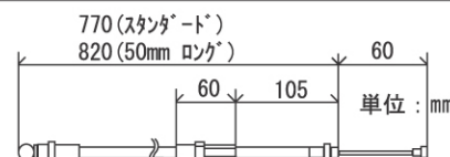
クラッチケーブル寸法図
