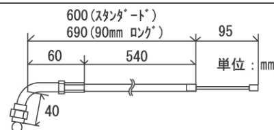
スロットルケーブル寸法図
