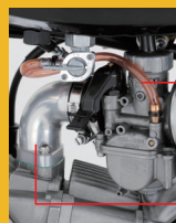
900222: ケイビンPE22 キャブレターASSY ¥14,175 (税込)
